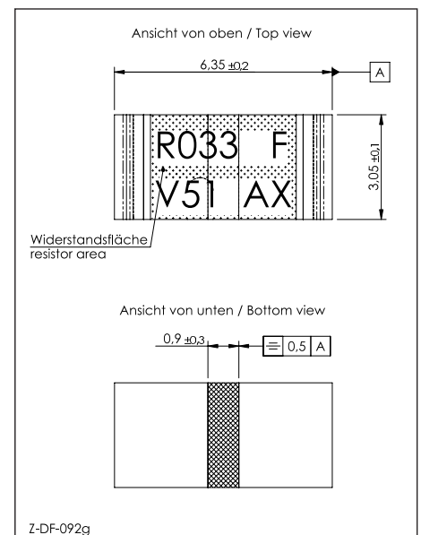
Bauform / Size 2512
